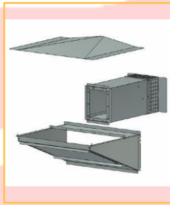
Zestaw do montażu na zewnątrz
